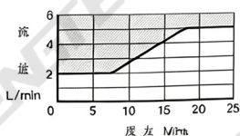
最小流量特性
