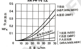
压降特性
