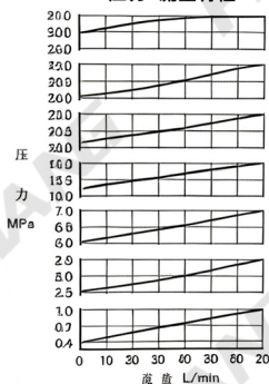
压力-流量特性
