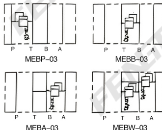
液压符号
