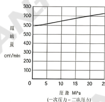
泄油量特性
