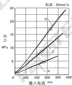
输入电流-压力特性
