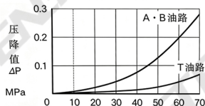
各油路压力特性
