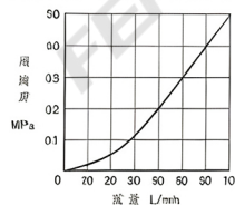
阀芯全开时的压降特性(P油路)
