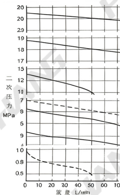
流量-压力特性 一次压力25MPa
