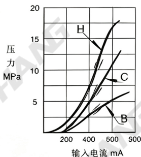
输入电流-压力特性
