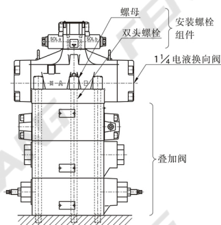
10系列叠加阀装配例
