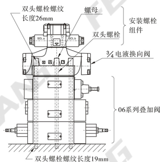
06系列叠加阀 装配例
