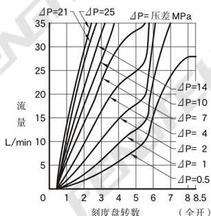
开度—流量特性
