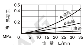
各油路压降特性
