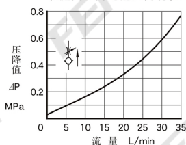
各油路压降特性
