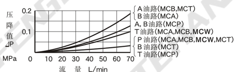
各油路压降特性
