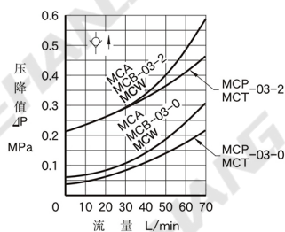
自由流压降特性
