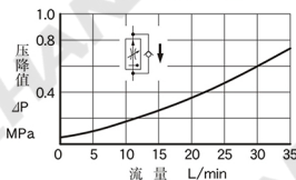
自由流压降特性
