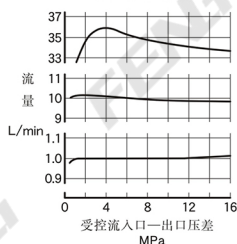
压力流量特性
