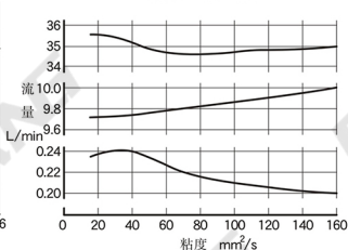
自由流压降特性
