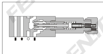
JIS液压图形符号
