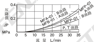
各油路压降特性
