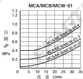
各油路压降特性
