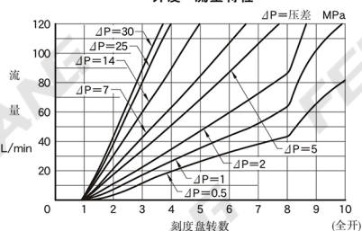
开度—流量特性
