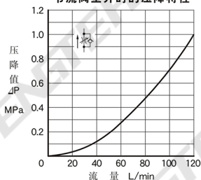
节流阀全开时的压降特性
