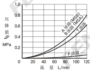
自由流压降特性
