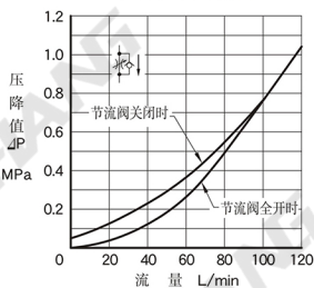
节流阀全开时的压降特性
